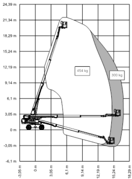
S-65 XC és S-65 TRAX mozgástartomány-diagramja
