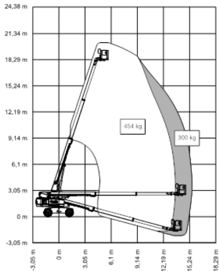
S-65 XC és S-65 TRAX mozgástartomány-diagramja
