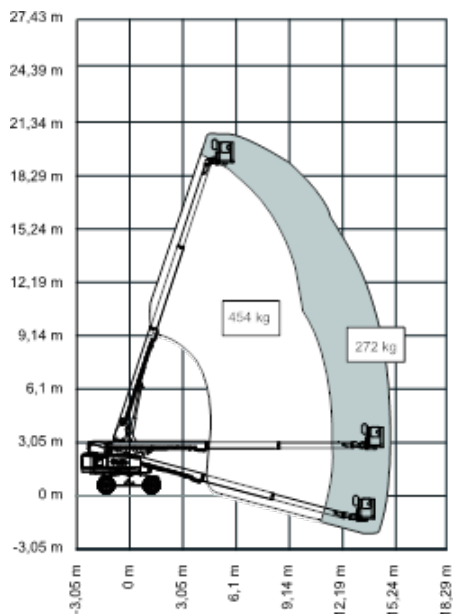
S-65 HF mozgástartomány-diagram
